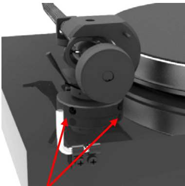
Madenschrauben
